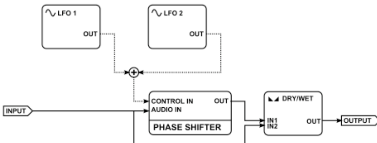
Écoulement du signal.
